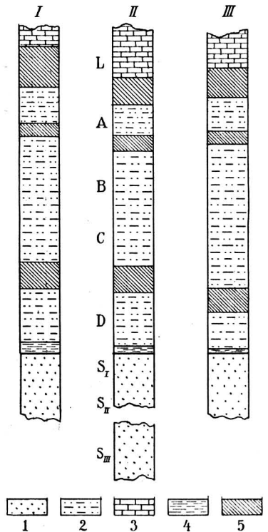
Fig. 5. Grænsezonen mellem Senon og Danien ved Voxlev.
