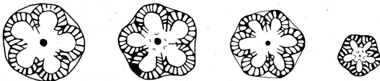
Fig. 9. Pentacrinus paucicirrhus Br. N.? Ledflader. Lag A, Voxlev. \frac{5}{1} .
