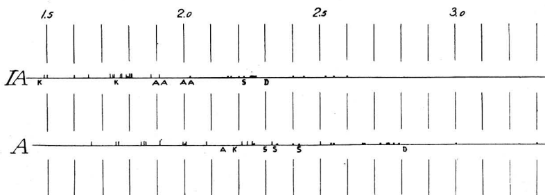
Fig. 10. Forholdet mellem Pladernes Bredde og Højde hos en Serie Echinocorys .
