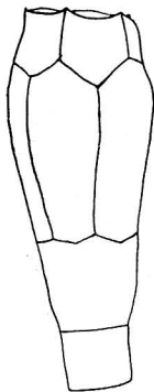
Fig. 8. Bourgueticrinus Brünnichi Nielsen n. sp. Lag B, Voxlev. 10/11.
