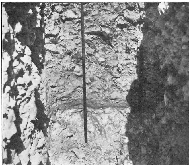
Fig. 7. Nordlige Udgravning (Profil III). Nederst Skrivekridt, derover med skarp Grænse Lerlaget, der foroven gaar over i »det døde Lag«.
